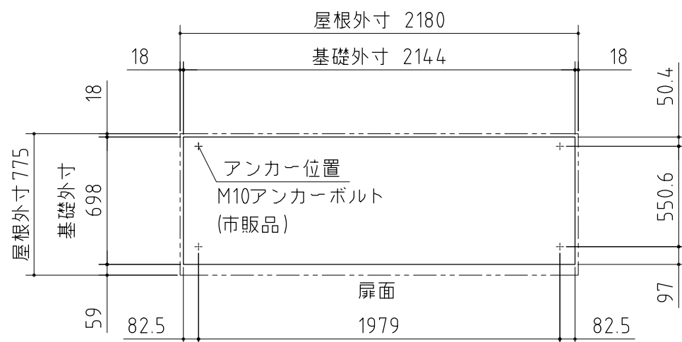
ベタ基礎図
